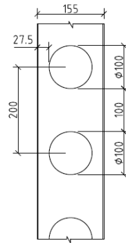
ELEVATION
